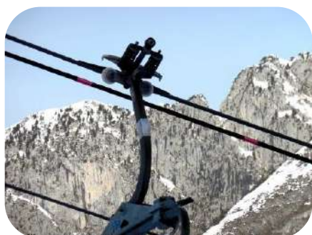
Inspection quinquennale des pinces du télésiège du Crêt-Béni
